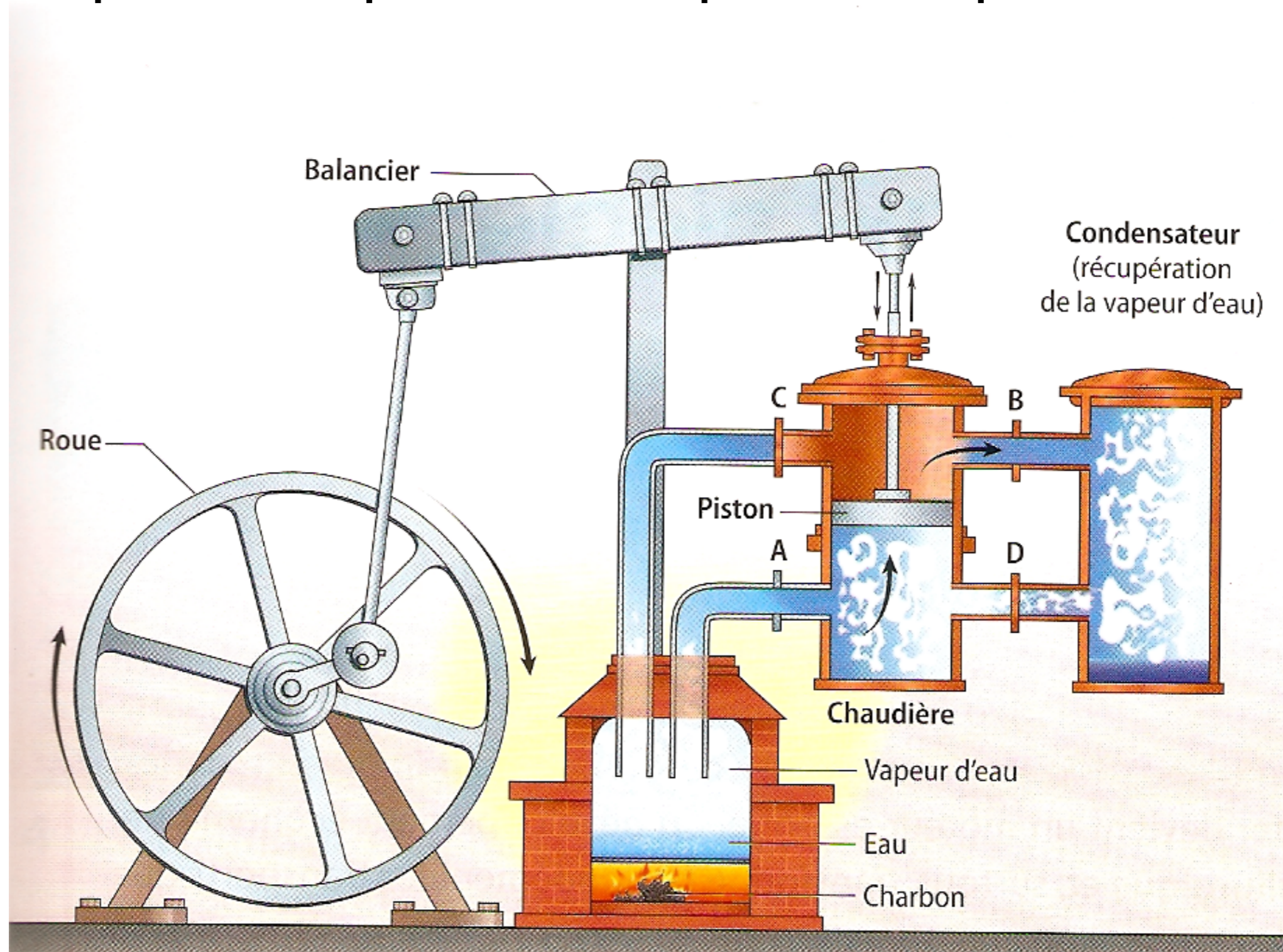
Machine à vapeur de James Watt. Angleterre (1780)
